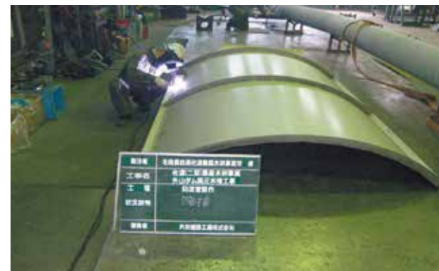
施設内防波管製作
