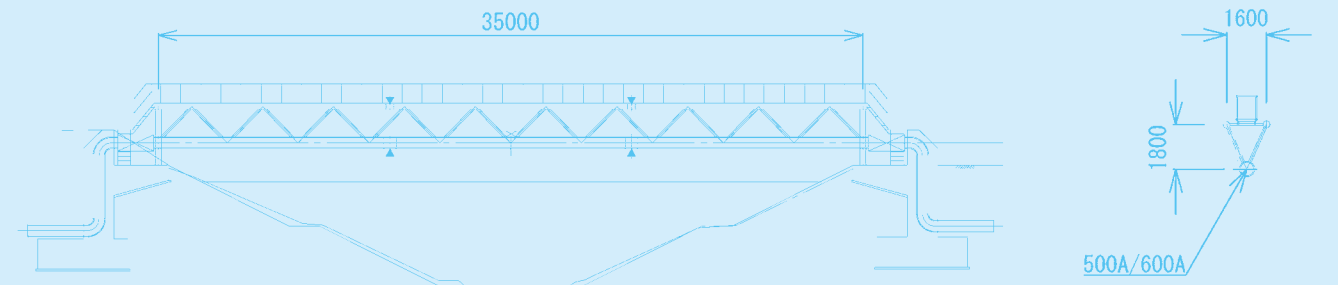
北海道石狩管内 新川水管橋 500A / 600A L=54.64m
