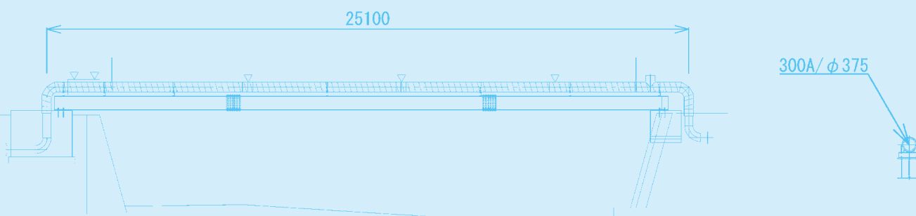
北海道渡島管内 板橋水管橋 300A / φ375 L=31.9m
