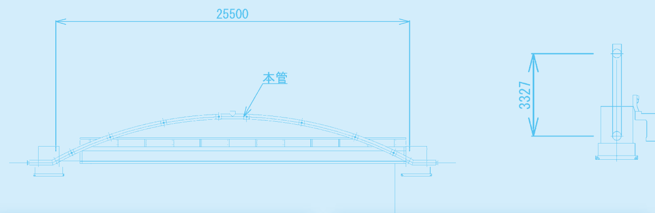
岩手県 神山橋 150A / 350A L=29.6m
